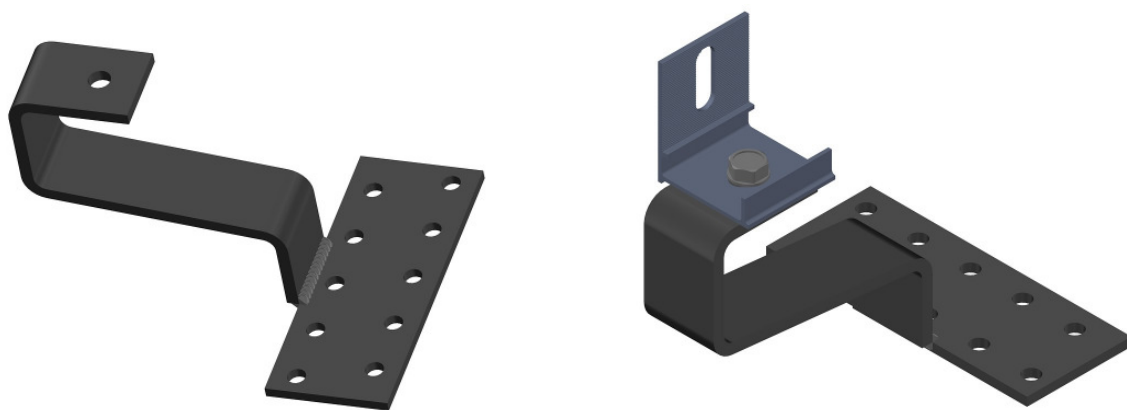
30 220 TS-Solar Edelstahldachhaken mit 30 203 Halterungswinkel und 30 210 Spermutter
