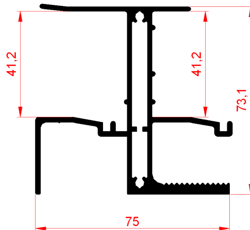
30 1045 Moduleinlegeschiene 40 mm
